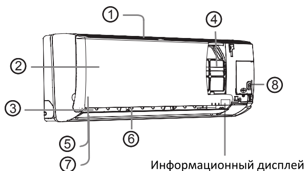
Внутренний блок
